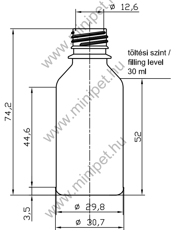
kupak nélkül / without cap
