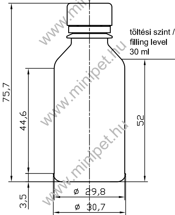
SK16 garanciazáras kupakkal / with Sk16 tamper evident cap
