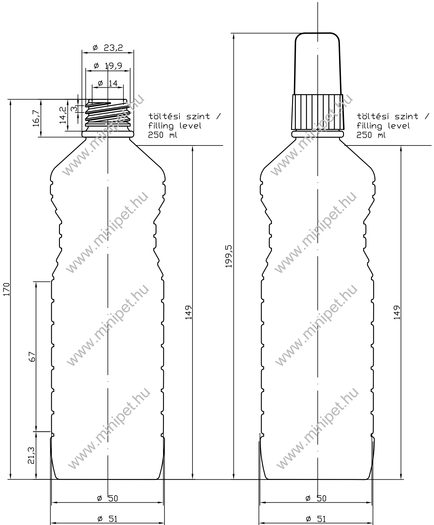
Termék/Product: PET palack/bottle Típus/Type: Olaj250 Menet/Neck: KS20G Súly/Weight: 17,5 gramm www.minipet.hu
